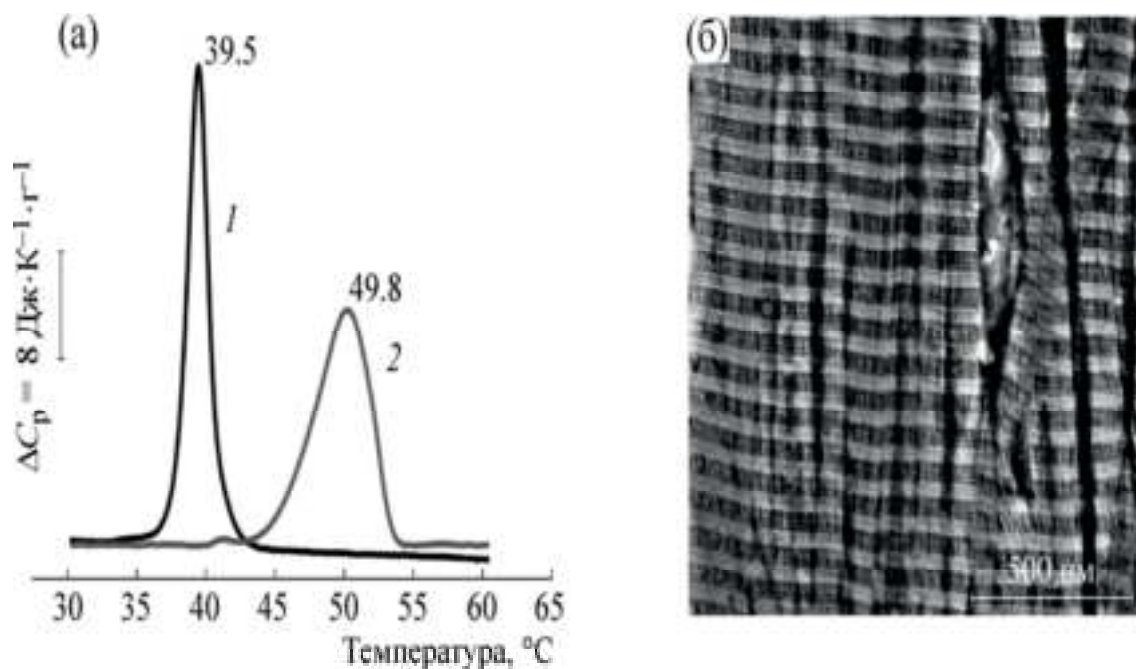
Рисунок 4. Характеристика формирующихся фибрилл. (а) – Термограммы плавления: 1 – мономерная форма коллагена в 0,2 М уксусной кислоте; 2 – фибриллярная форма коллагена в фосфатно-солевом буфере; (б) – микрофотография образца коллагена (фибриллярная форма)
