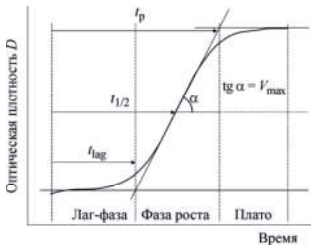
Рисунок 2. Схема измерения параметров кривых светорассеяния, представленных на рис. 3. Показано измерение длительности лаг-фазы ( t_{lag} ), времени достижения половины максимального роста ( t_{1/2} ), времени достижения плато на кривой светорассеяния ( t_p ), а также определение величины максимальной скорости роста светорассеяния ( V_{max} ).
