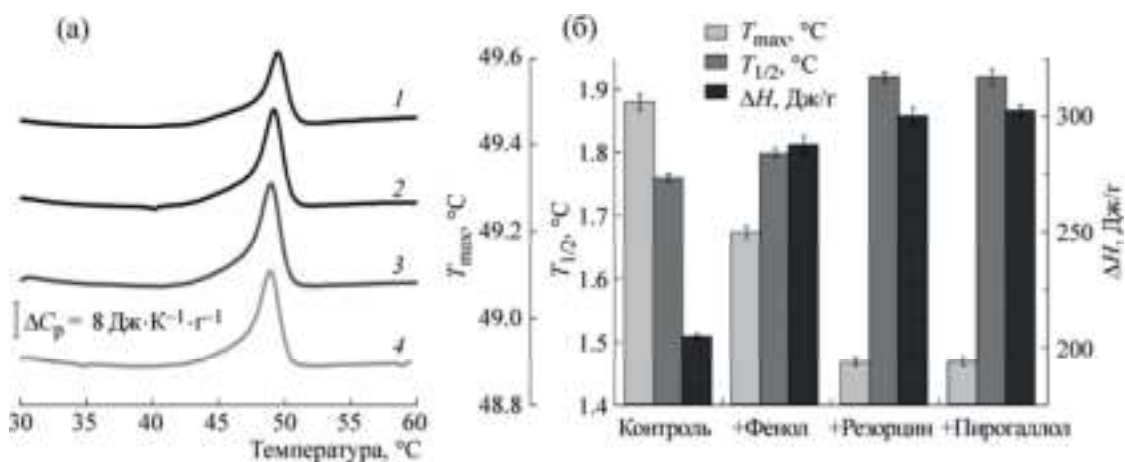
Рисунок 5. Влияние фенолов на термические характеристики формирующихся фибрилл. (а) – Термограммы плавления фибрилл коллагена: 1 – коллаген, 0,2 мг/мл; 2 – в присутствии фенола; 3 – в присутствии резорцина; 4 – в присутствии пирогаллола. Концентрация фенолов во всех экспериментах составляла 10 мкМ. (б) – Параметры термограмм, представленных на рис. 5а.
