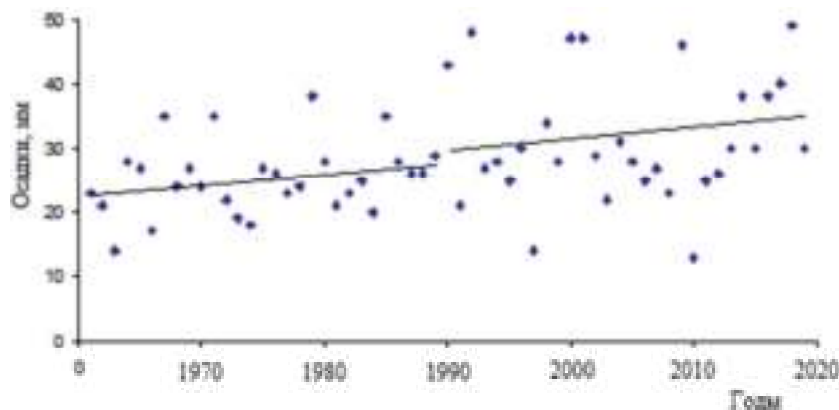
Рисунок 7. Временной ход средних показателей осадков за теплый период (апрель-октябрь) с 1961 по 2019 гг.
