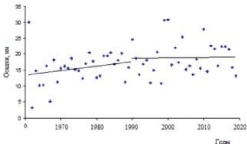
Рисунок 8. Временной ход средних показателей осадков за холодный период (ноябрь-март) с 1961 по 2019 гг.
