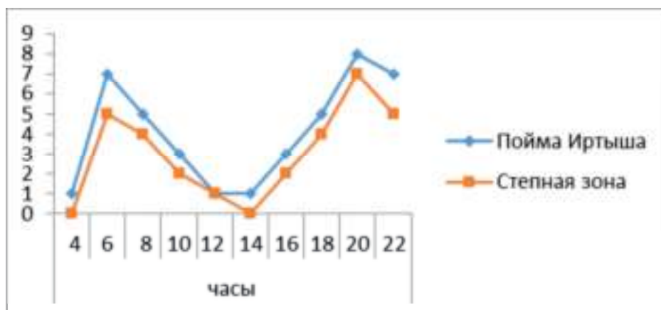
Рисунок 2. Суточная активность Anopheles messeae
