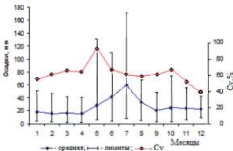
Рисунок 6. Характеристика осадков по месяцам в 1990-2019 гг.
