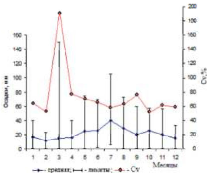
Рисунок 5. Характеристика осадков по месяцам в 1961-1989 гг.
