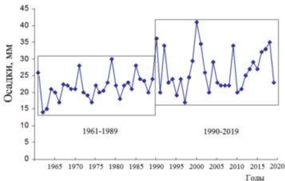
Рисунок 4. Временной ход среднегодовых показателей осадков с 1961 по 2019 гг.
