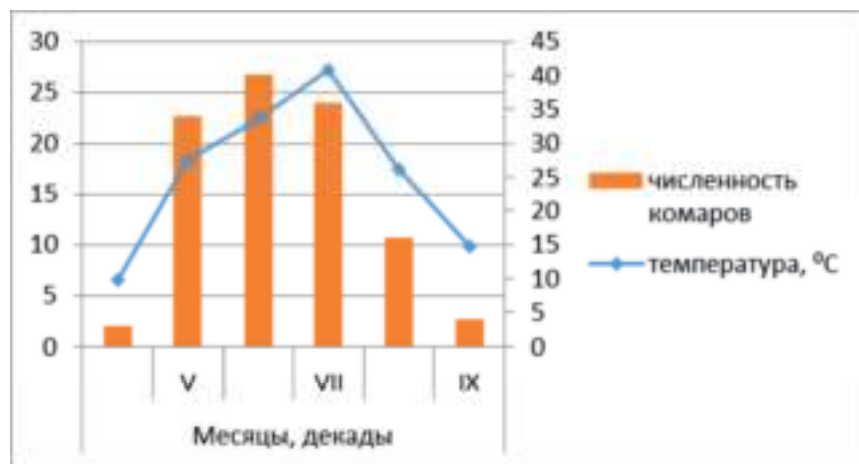
Рисунок 1. Сезонный ход численности Anopheles messeae
