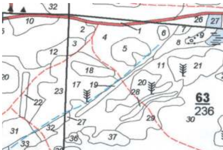
Рисунок 13. Картографическое расположение мониторинговых площадок №7 (Баянаульское подразделение) квартал 63, 12 - выдел.
